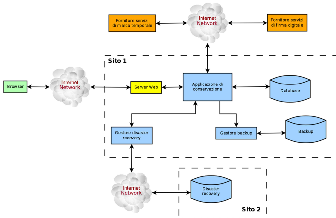
Figura 10 - Schema componenti del Servizio
