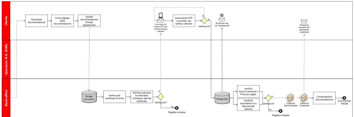
Figura 11 - Flusso di rilascio Identità Digitale per persona giuridica con identificazione mediante dispositivo di firma elettronica qualificata o digitale
