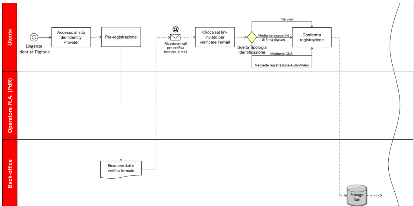
Figura 5 - Flusso di Pre-registrazione
