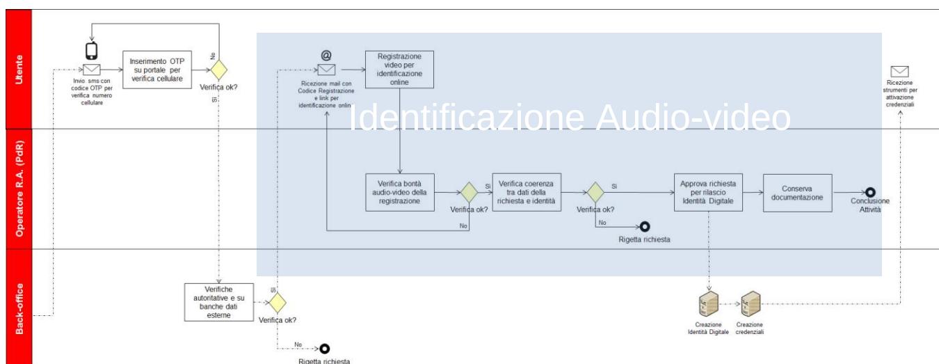
Figura 13 - Flusso di rilascio Identità Digitale per persona giuridica con identificazione Audio-Video
