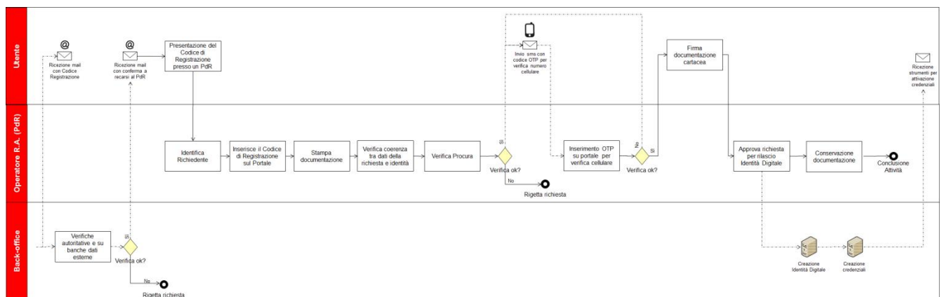
Figura 10 - Flusso di rilascio Identità Digitale per persona giuridica con identificazione 'De Visu'
