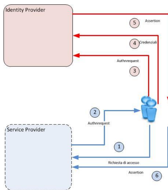
Figura 4 – Flusso di autenticazione utente
