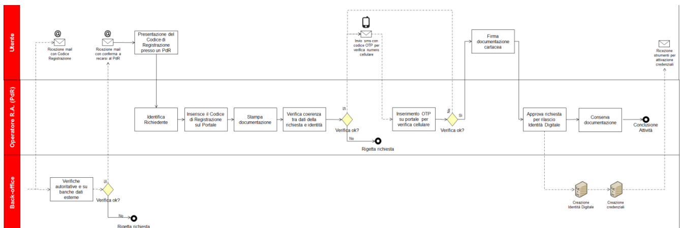
Figura 6 - Flusso di rilascio Identità Digitale per persona fisica con identificazione 'De Visu'
