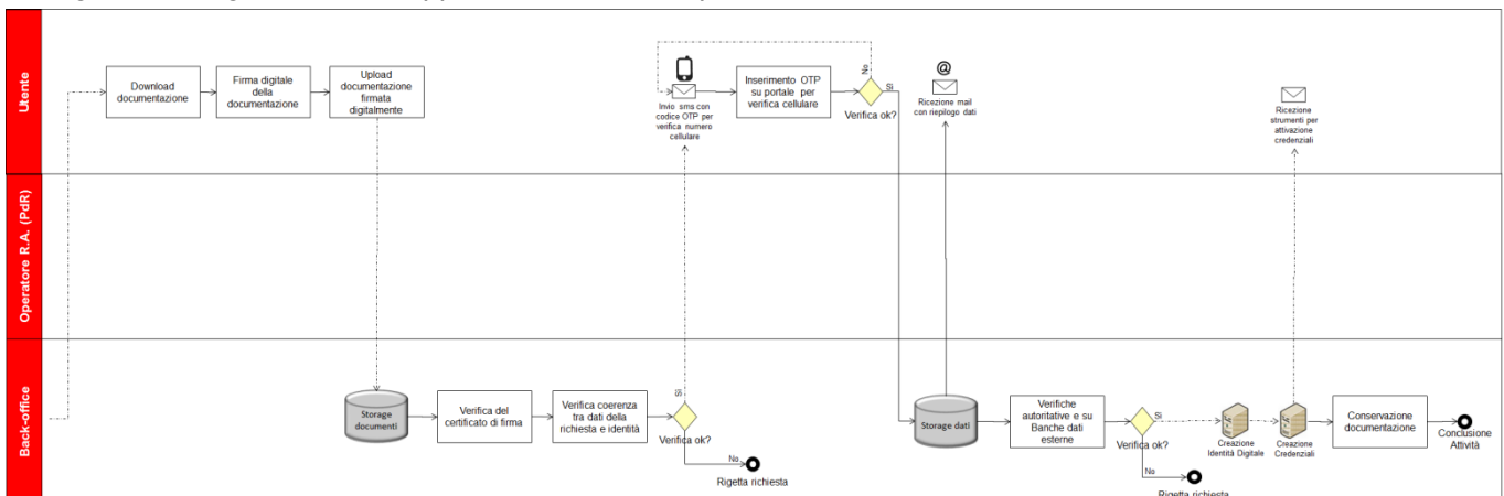
Figura 7 - Flusso di rilascio Identità Digitale per persona fisica con identificazione mediante dispositivo di firma elettronica qualificata o digitale
