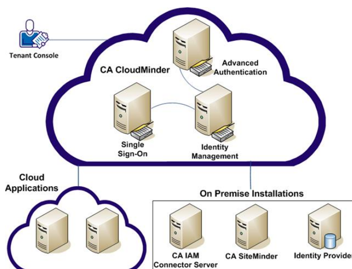
Figura 1 – Architettura logica della piattaforma
