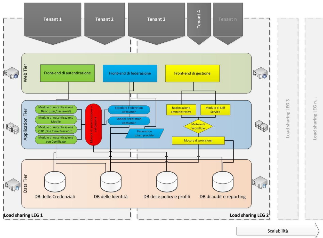
Figura 2 – Architettura 3-Tier (a 3 livelli) della piattaforma
