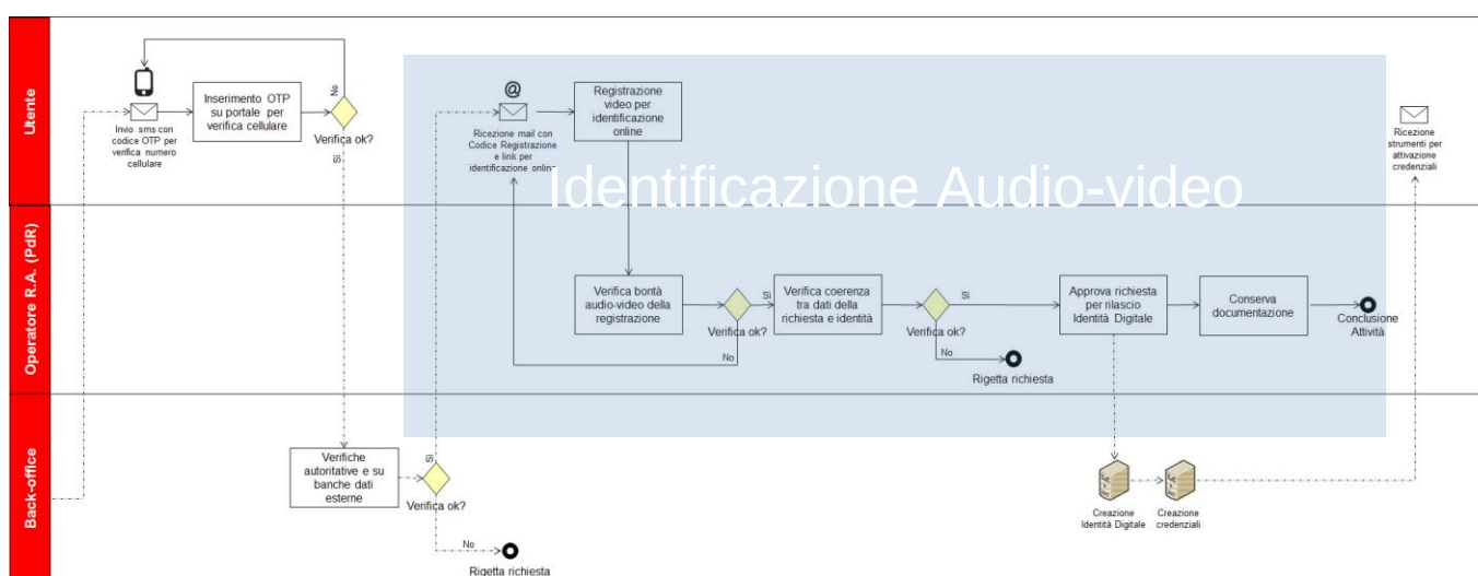
Figura 9 - Flusso di rilascio Identità Digitale per persona fisica con identificazione Audio-Video
