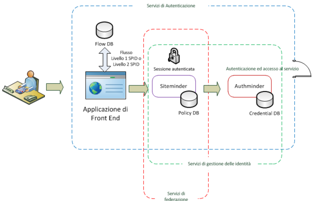
Figura 3 – Schema dei servizi di autenticazione
