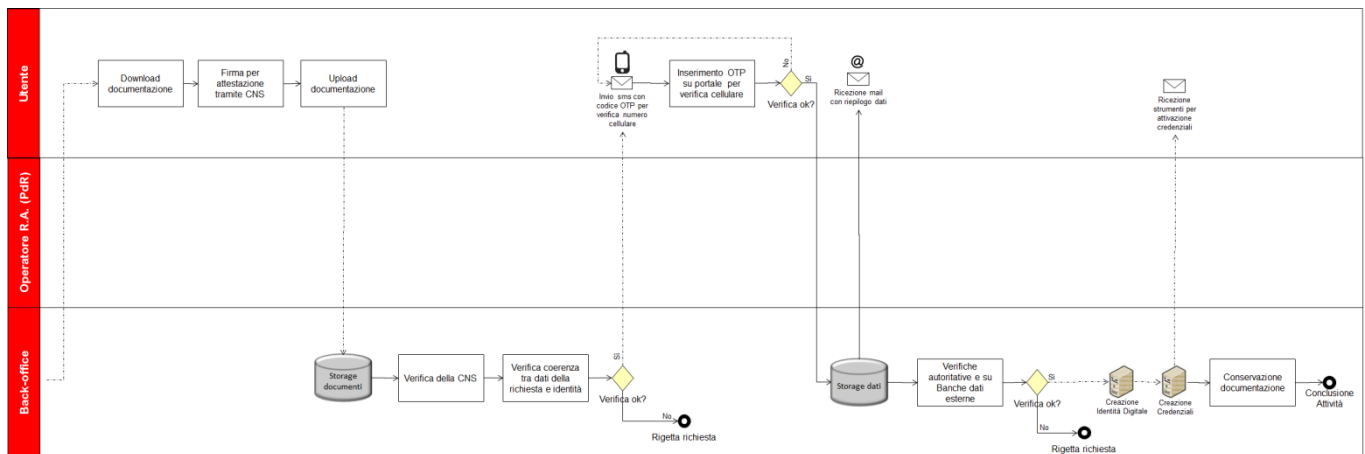
Figura 8 - Flusso di rilascio Identità Digitale per persona fisica con identificazione mediante utilizzo di CNS e CIE
