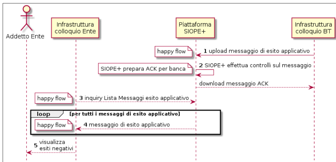
Figura 21 - Sequence diagram del processo di scambio del messaggio di esito applicativo
