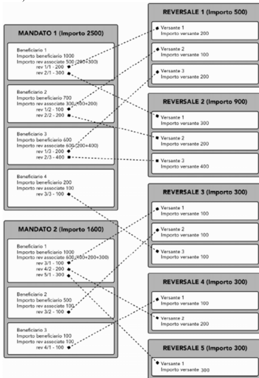
Figura 8 - Rappresentazione grafica legami mandati / reversali
