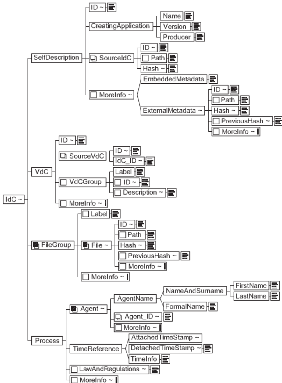
Figura 3: struttura dell'indice del pacchetto di archiviazione
