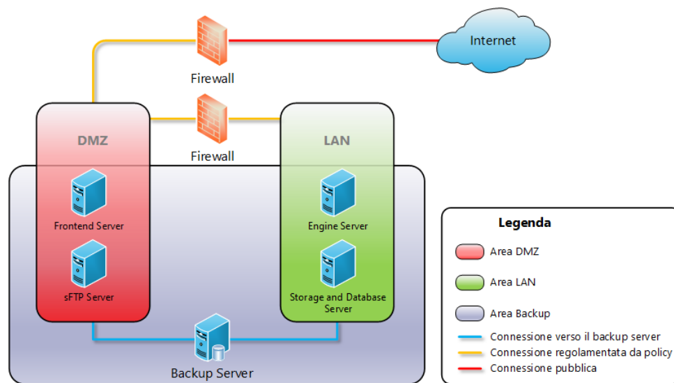
Figura 8: schema dell'infrastruttura della farm di produzione
