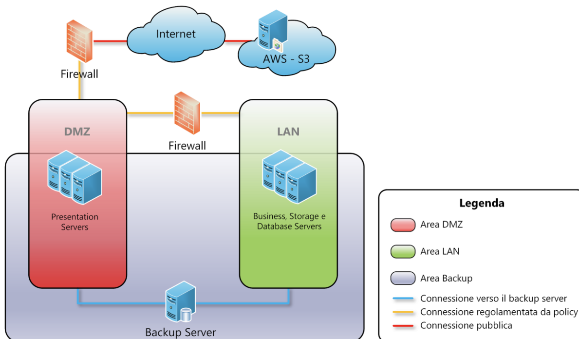
Figura 8: schema dell'infrastruttura della farm di produzione
