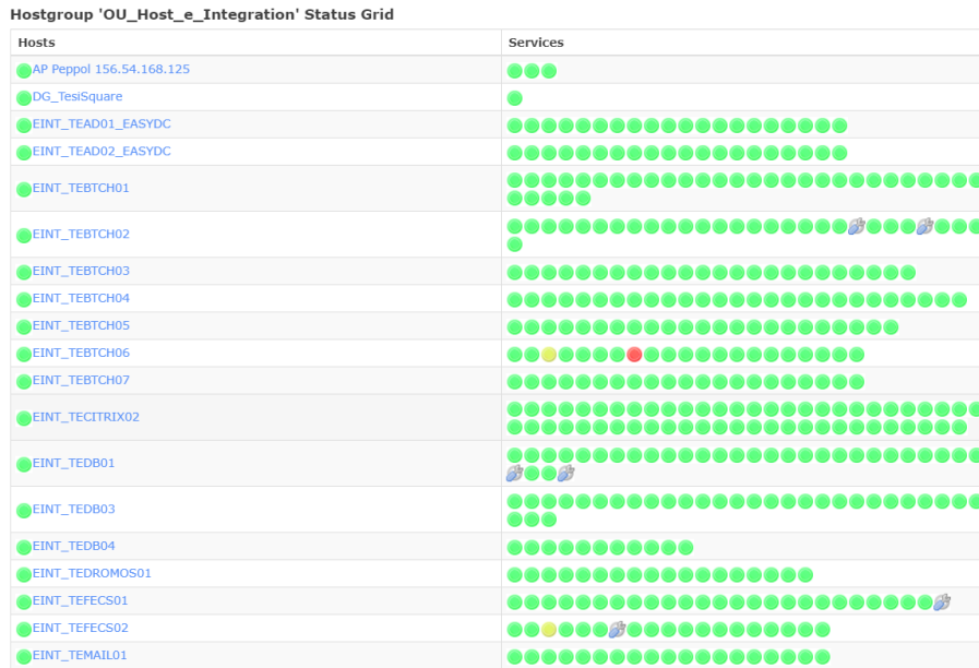
Figura 30. Schermata di controllo Nagios
