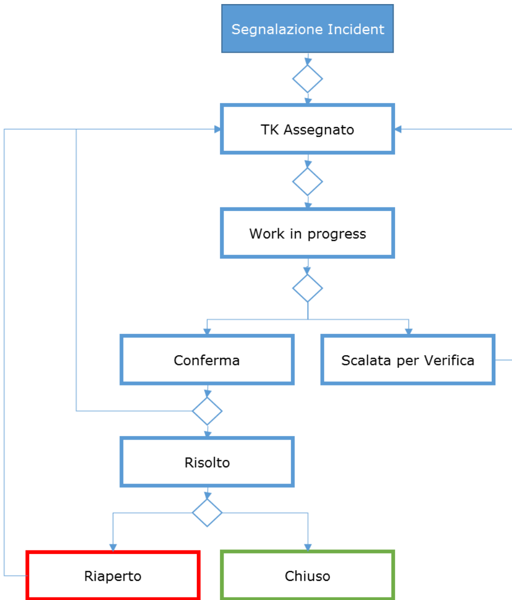
Figura 33. Gestione incident
