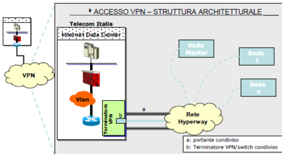
Figura 28. Struttura logica
