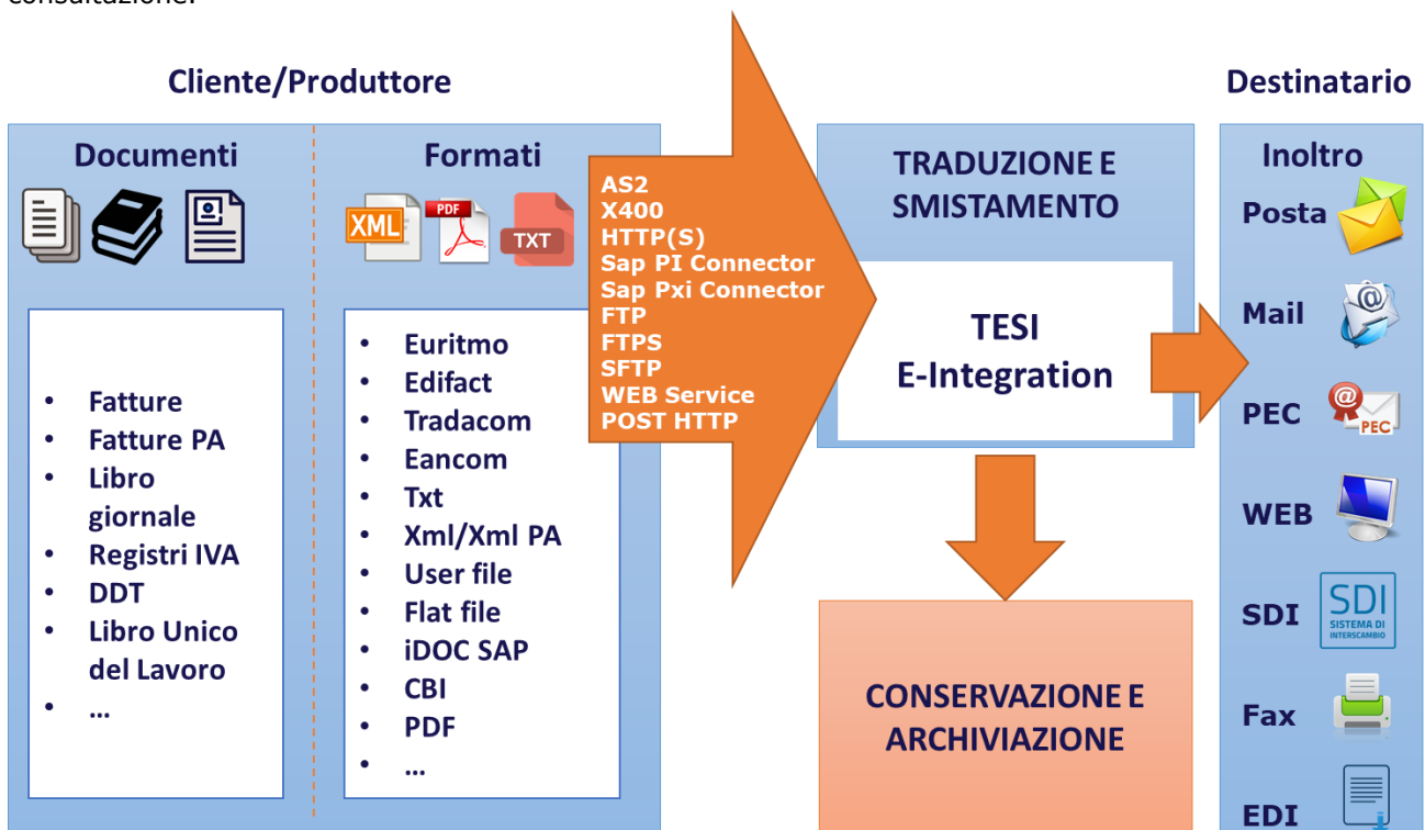
Figura 10. Multicanalità
