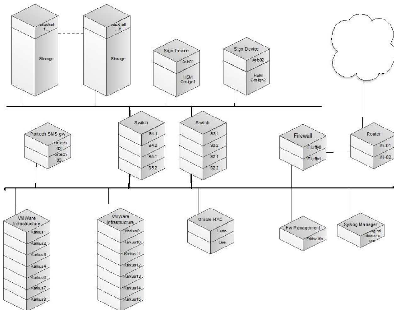
Figura 4. Architettura del sistema di conservazione (schema logico dei datacenter)
