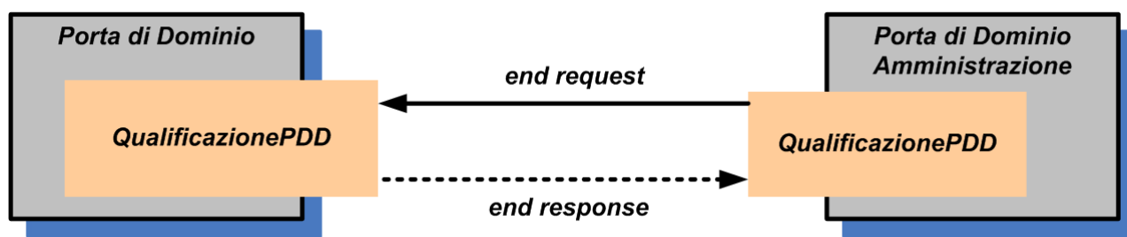
Fig 59. Caso di Test: end
