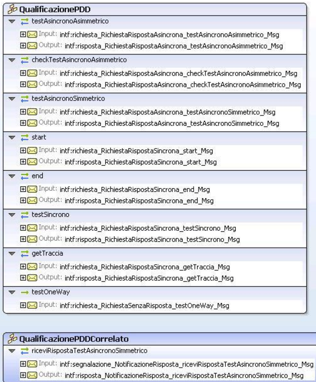
Fig 1. Rappresentazione grafica del WSDL Concettuale
