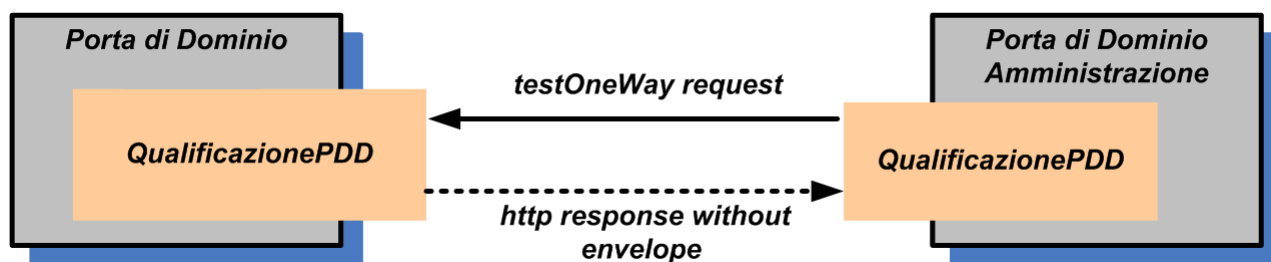
Fig 42. Caso di test: testOneWay
