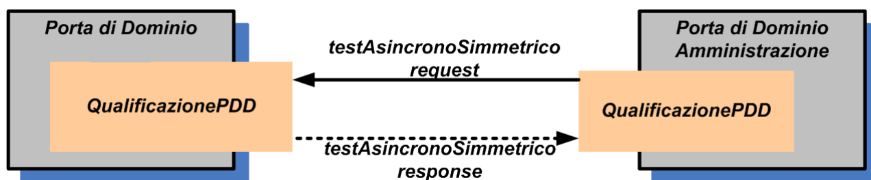
Fig 53. Caso di Test: testAsincronoSimmetrico
