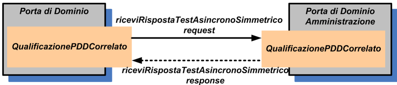
Fig 54. Caso di Test: riceviRispostaTestAsincronoSimmetrico
