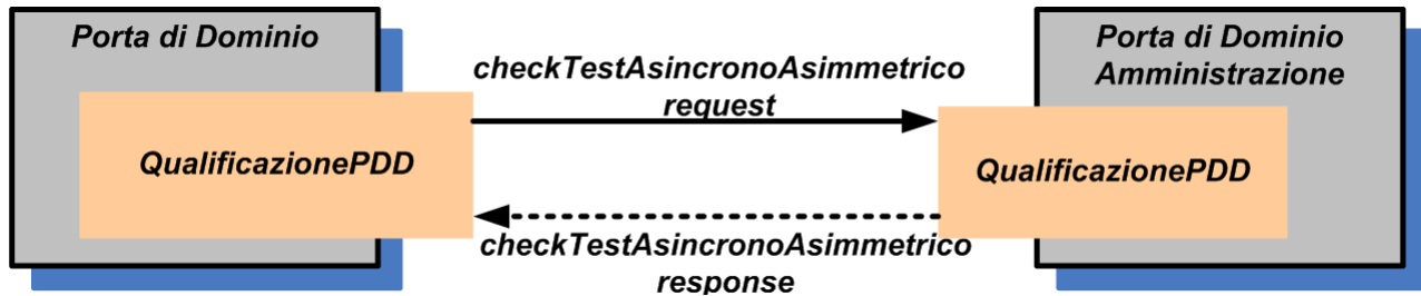
Fig 25. Caso di Test: checkTestAsincronoAsimmetrico
