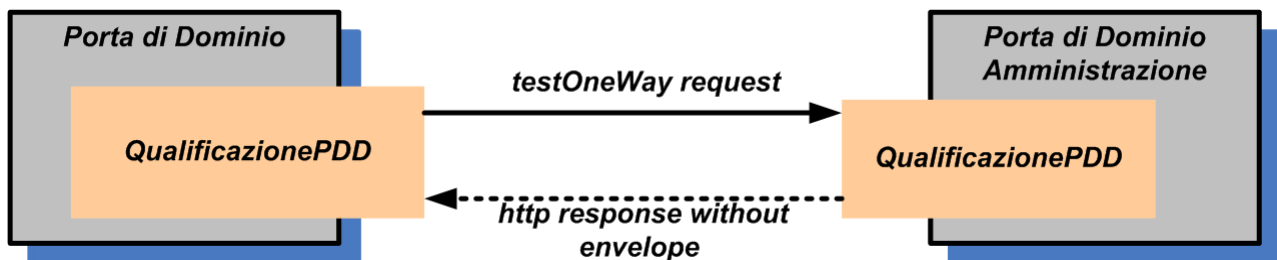
Fig 19. Caso di Test: testOneWay
