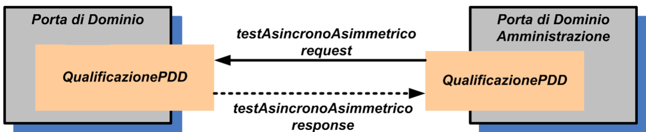
Fig 47. Caso di Test: testAsincronoAsimmetrico
