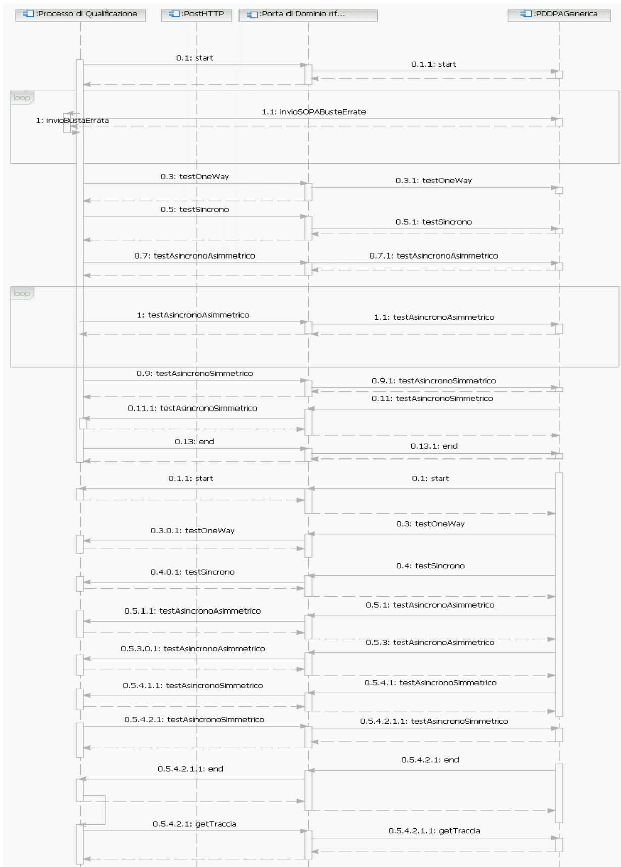
Fig 6. Sequence Diagram delle operazioni di test
