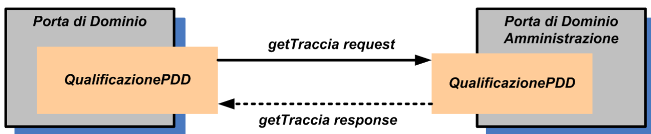
Fig 62. Caso di Test: getTraccia.
