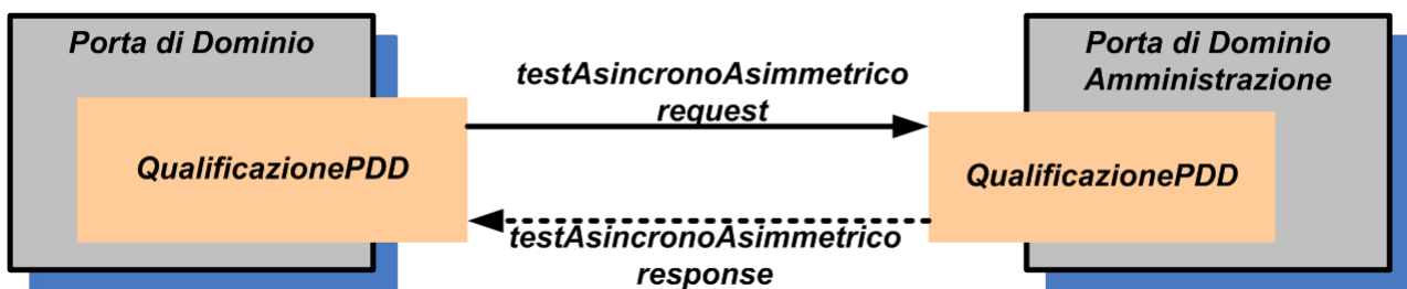
Fig 24. Caso di Test: testAsincronoAsimmetrico
