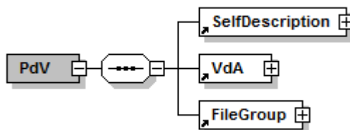
Fig. 1 - Struttura Indice PdV: suddiviso in SelfDescription, VdA e FileGroup
