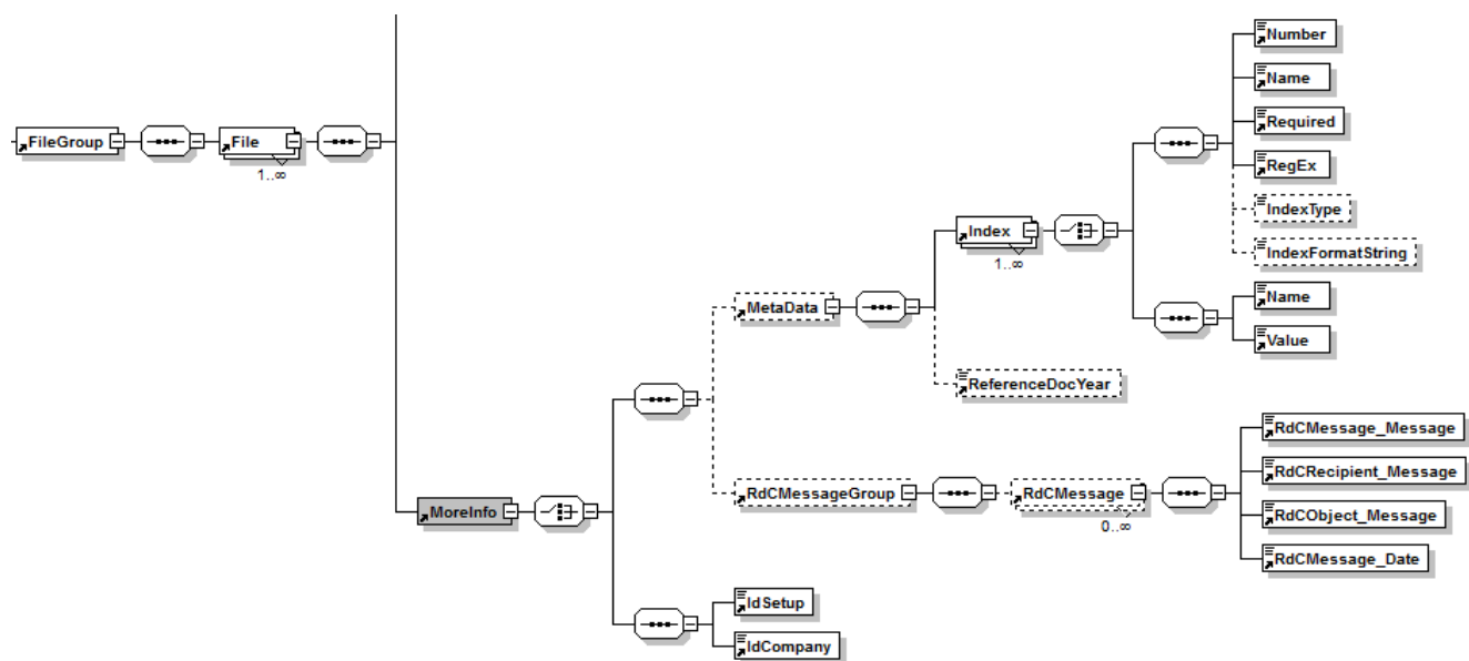
Fig. 4 - Struttura Indice PdV (Sezione FileGroup)
