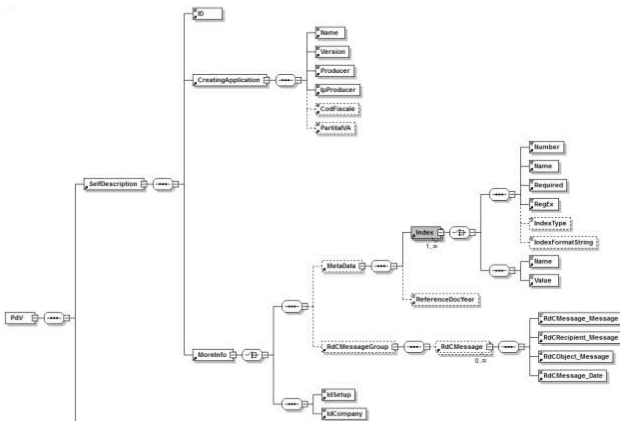
Fig. 2 - Struttura Indice PdV (Sezione SelfDescription)
