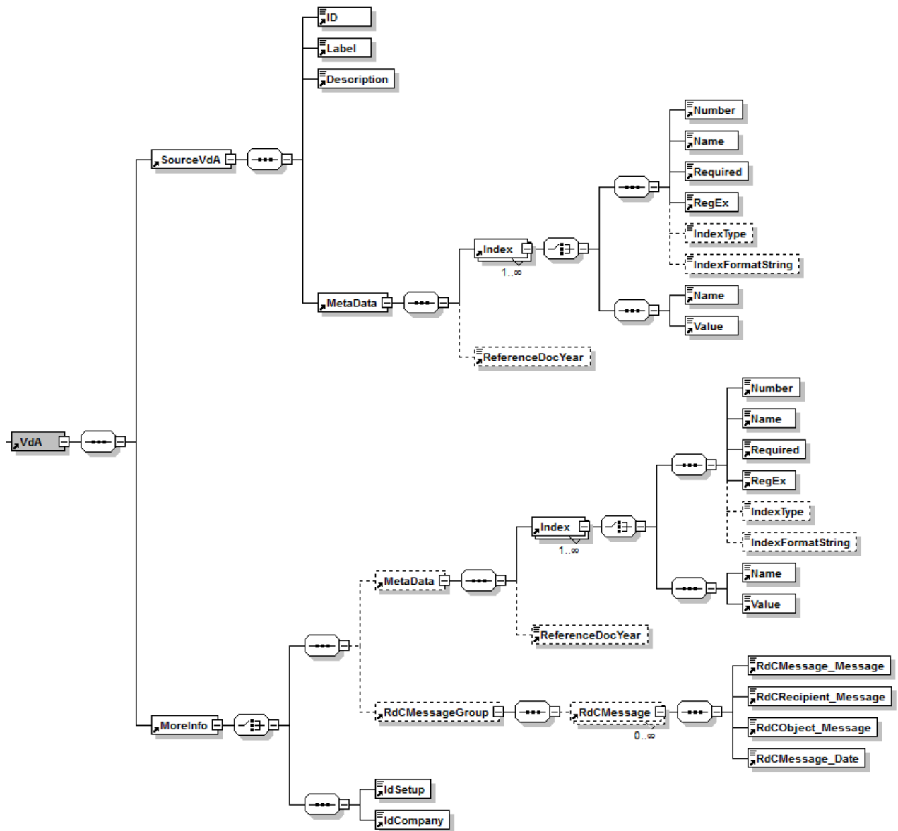
Fig. 3 - Struttura Indice PdV (Sezione VdA)
