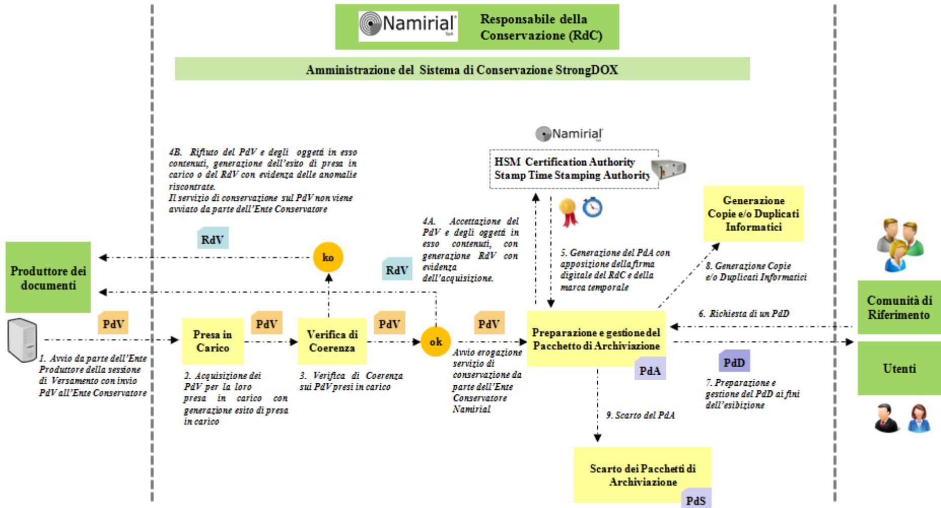
Fig. 5 – Processo di conservazione in Strongdox
