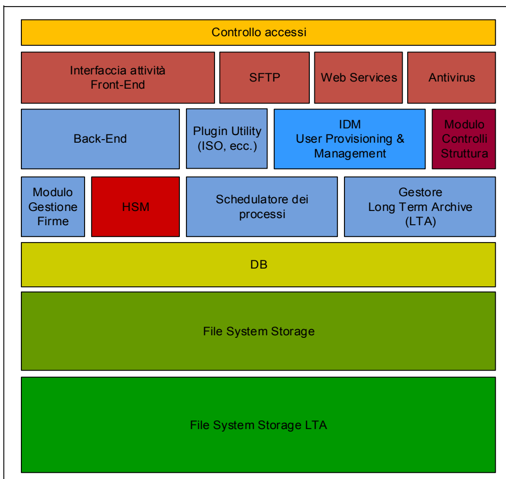
Fig. 6 - Componenti del sistema di conservazione Strongdox
