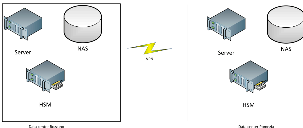
Figura 4 - Componenti fisiche
