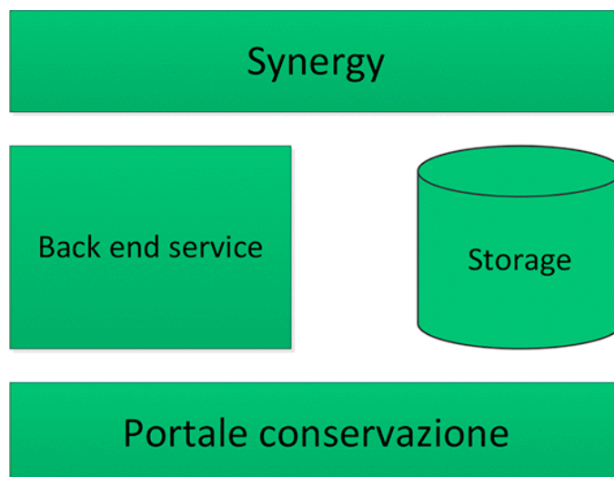
Figura 2 - Componenti logiche
