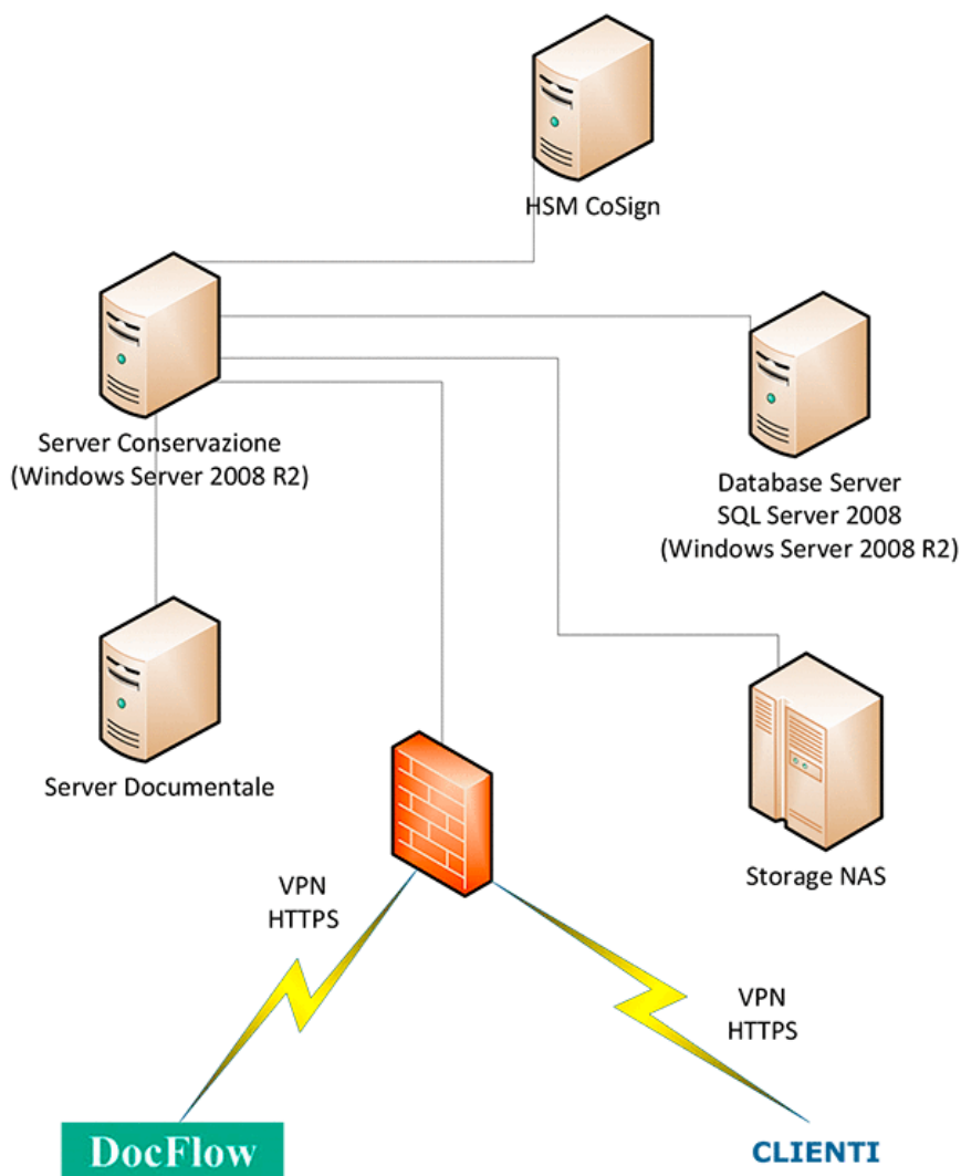
Figura 3 - Componenti tecnologiche
