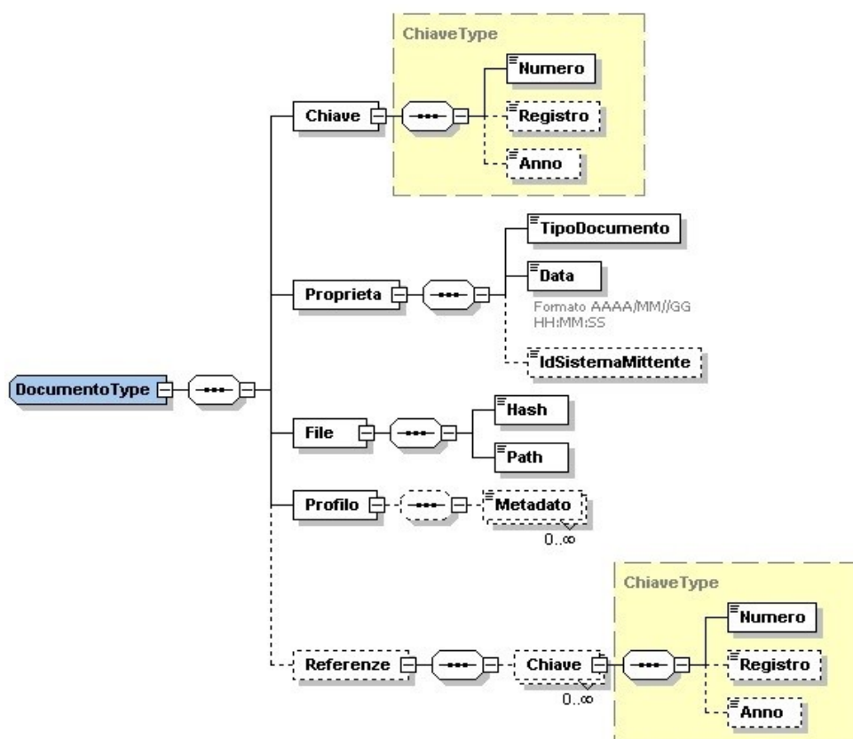
Figura 3 - Nodo documento
