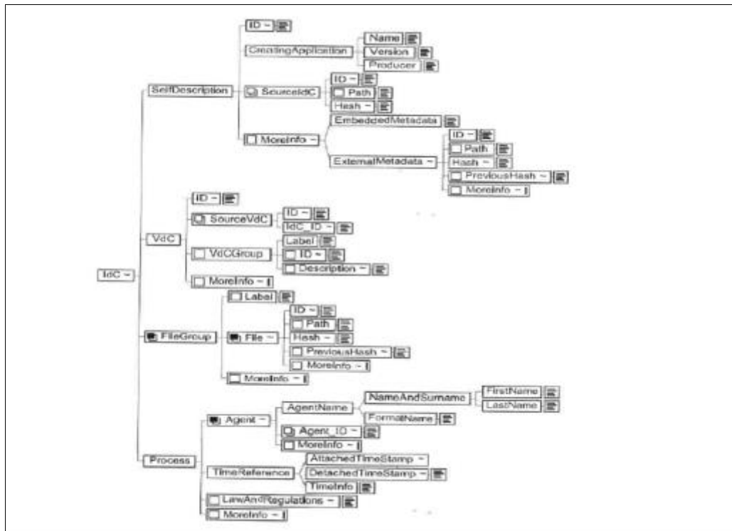
Figura 7:Struttura pacchetto di archiviazione secondo lo standard UNI 11386
