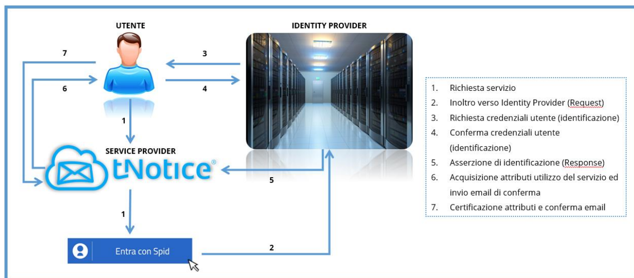
Schema registrazione utente
