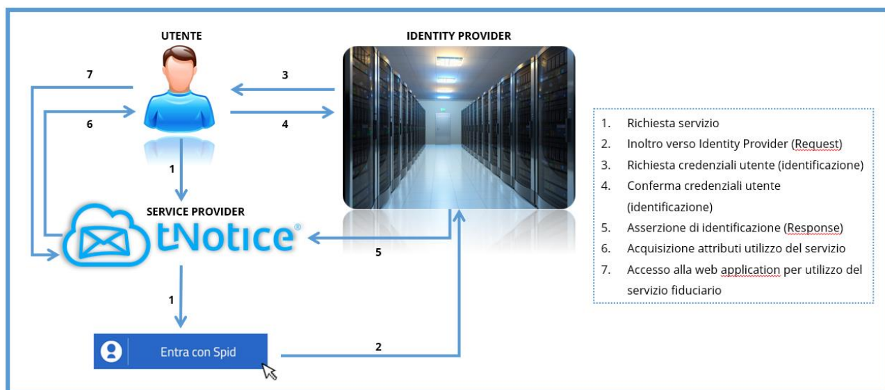
Schema accesso utente
