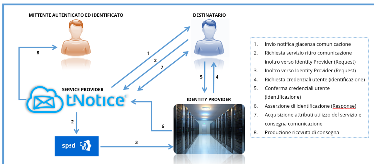
Schema processo di notifica, identificazione destinatario e consegna comunicazione
