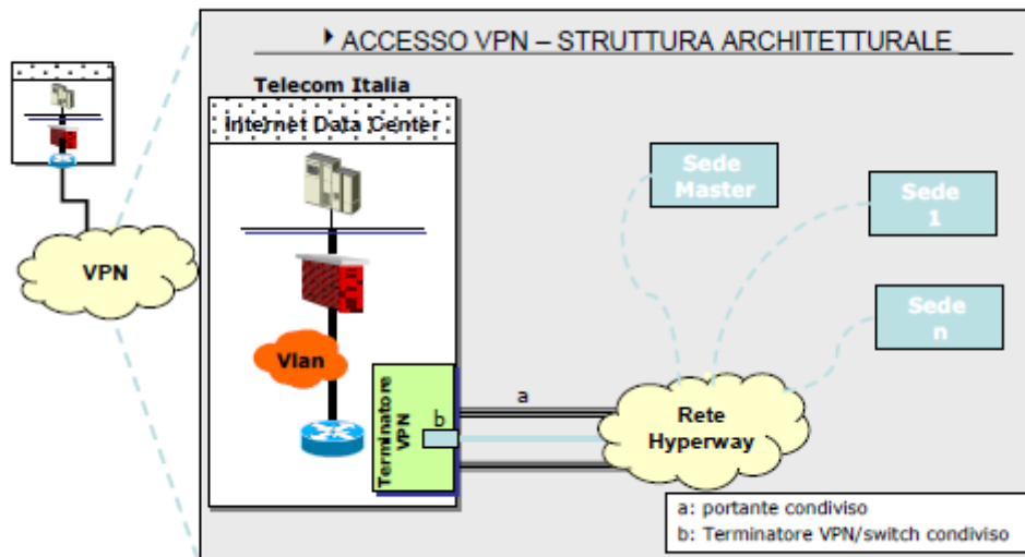
Figura 28. Struttura logica
