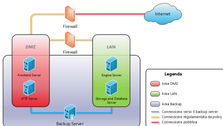
Figura 8: schema dell'infrastruttura della farm di produzione
