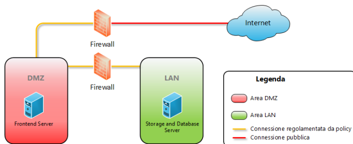
Figura 9: schema dell'infrastruttura della farm di DR
