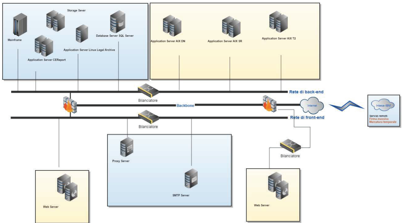
Figura 12. Infrastruttura generale.
