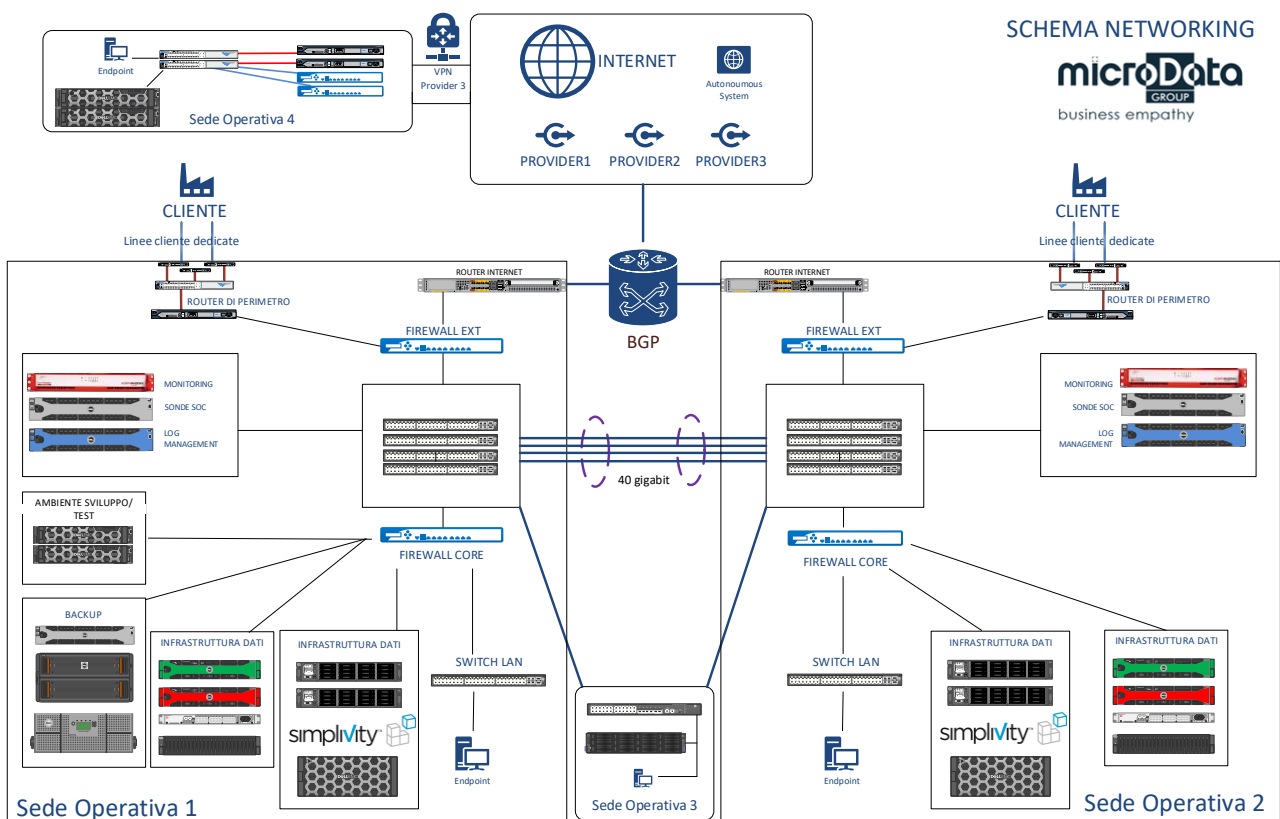
Figura 10: Schema di rete di Microdata
