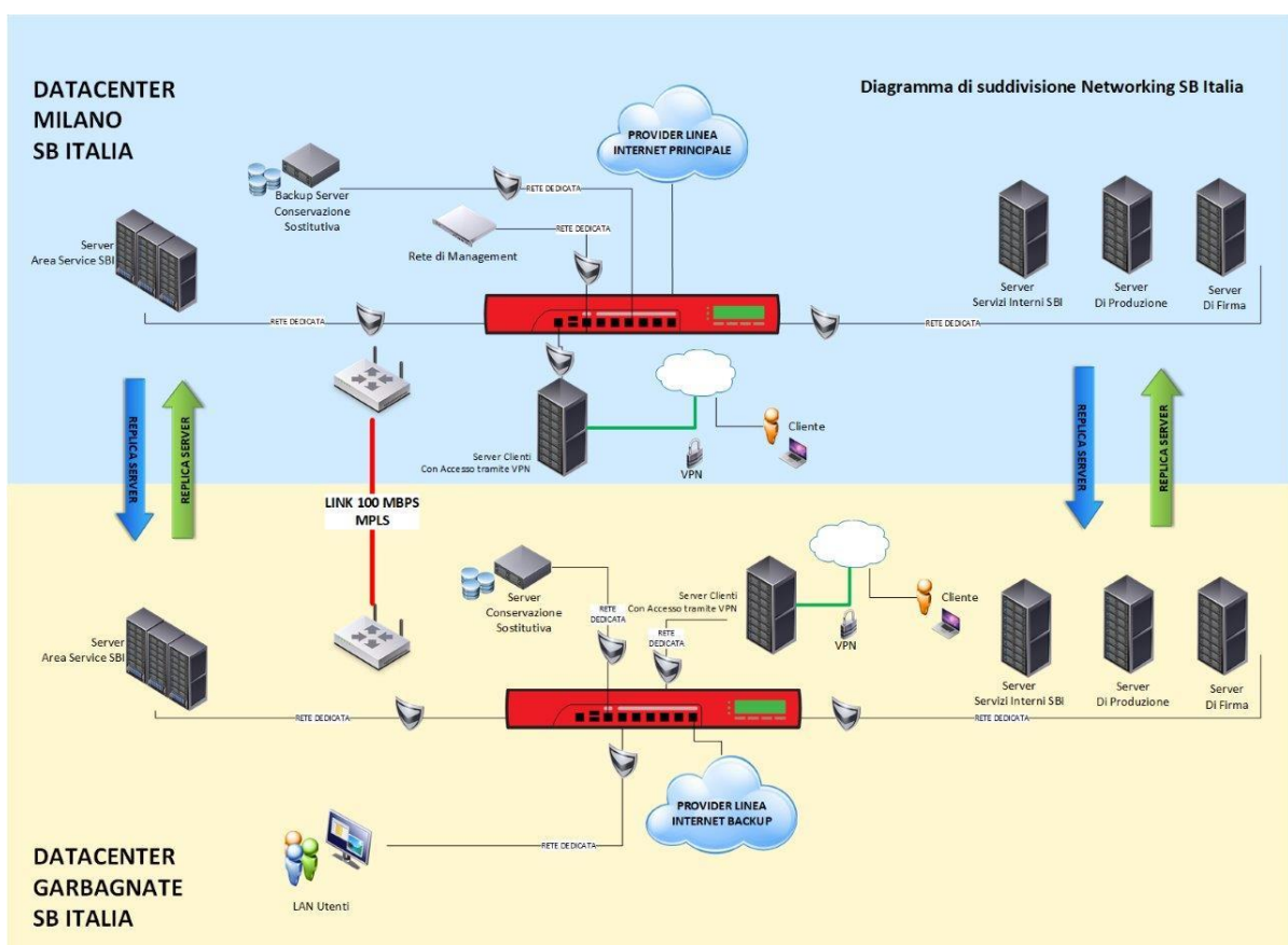
Figura 9 Schema Infrastruttura
