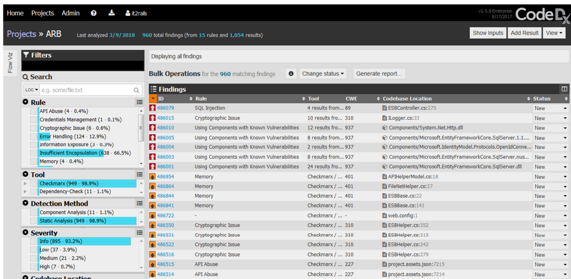
Figura 22 - Interfaccia CodeDx
