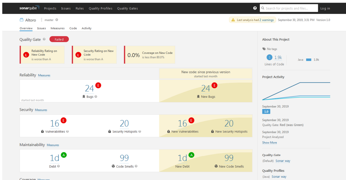
Figura 24 - SonarQube
