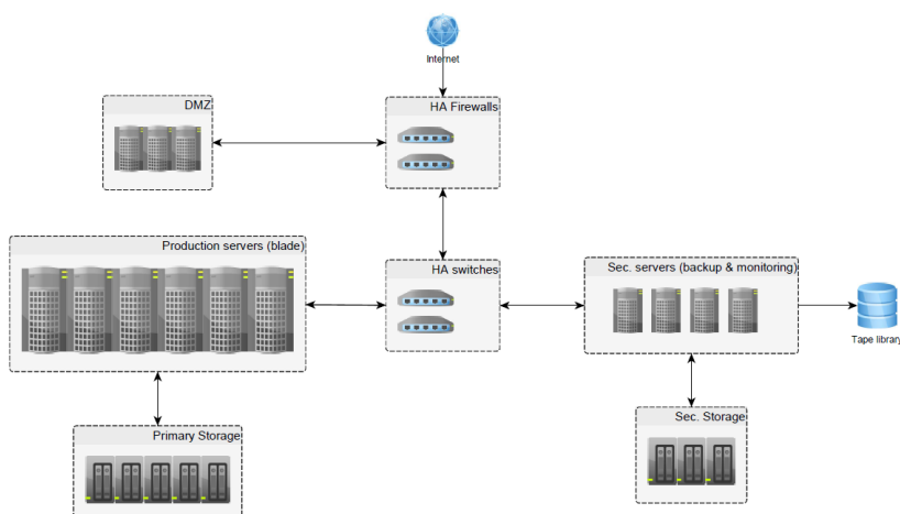
Figura 6. Architettura implementata da Faber System
