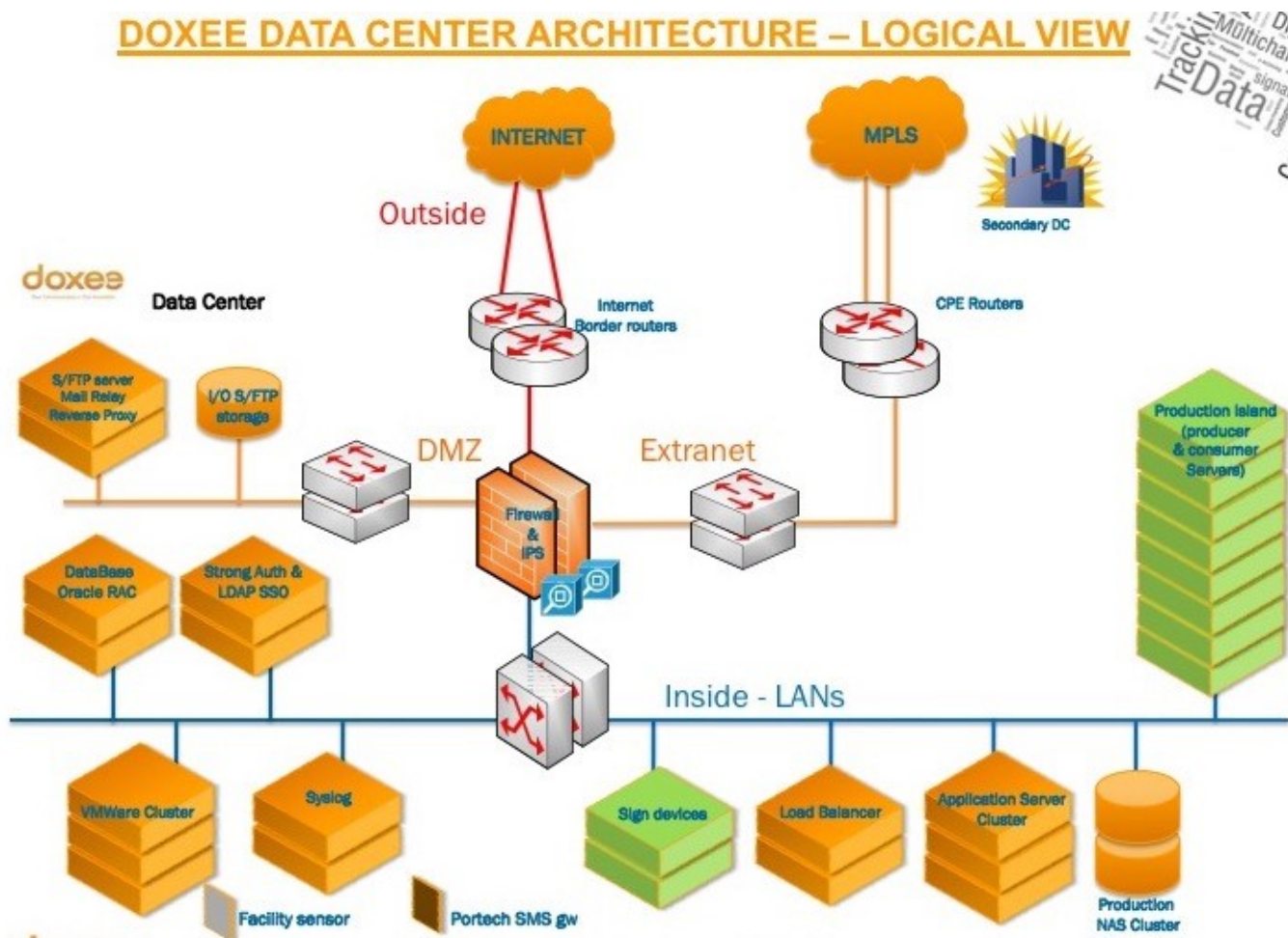
Figura 4. Architettura del sistema di conservazione (schema logico dei datacenter)
